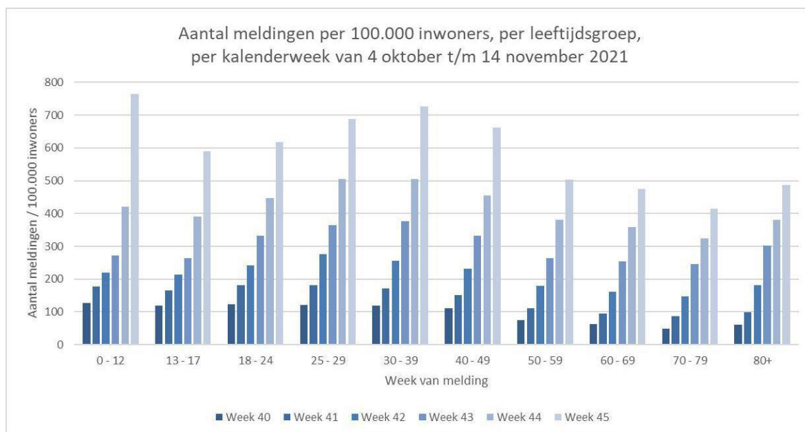
Figuur 1. Aantal COVID-19 meldingen per 100.000 inwoners, per leeftijdsgroep, per week van 4 oktober t/m 14 november 2021. Bron: RIVM (openbaar, nieuwsbericht).
