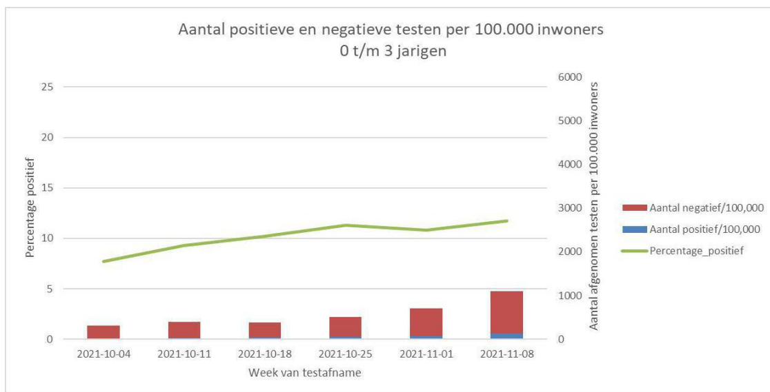
Figuur 3: Aantal positieve, negatieve en percentage positieve testen per week en per leeftijdsgroep vanaf 4 oktober. Op de linker y-as het percentage positieve testen, op de rechter y-as het aantal afgenomen testen per 100.000 inwoner, op de x-as de week van testafname. De groene lijn geeft het percentage positieve testen weer. Rood zijn negatieve testen, blauw positieve testen. Bron: RIVM
