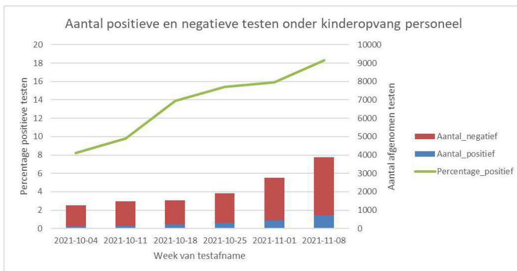
Figuur 5: Aantal positieve, negatieve en percentage positieve testen per week voor kinderopvang personeel vanaf 4 oktober. Op de linker y-as het percentage positieve testen, op de rechter y-as het aantal afgenomen testen per 100.000 inwoner, op de x-as de week van testafname. De groene lijn geeft het percentage positieve testen weer. Rood zijn negatieve testen, blauw positieve testen. Bron: RIVM.
